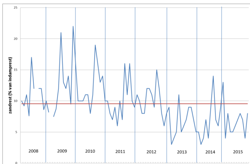
Afbeelding 2. Zandrest in de slibkoek van de svi Mierlo; periode 2008 – 2015
