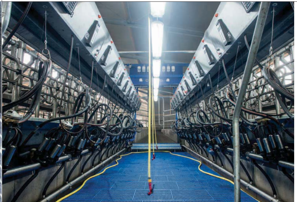
Links: de mest en het zand belanden achter de stal in een goot die wordt doorgespoeld met dunne fractie om mest en zand te scheiden Rechts: de koeien worden gemolken in een 2x12 zij-aan-zijstal met snelwisselsysteem
