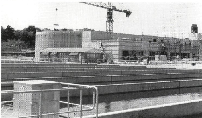
Voorbezinktanks en slibbehandeling (in aanbouw).
