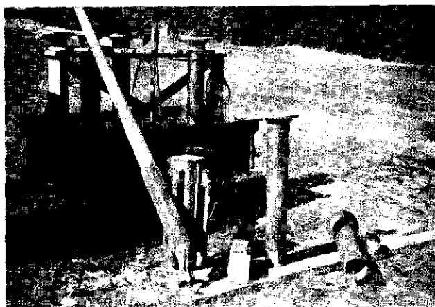
Afb. 2. Aanhangwagentje van de jeep, voor het vervoer van de stalen buizen en de nodige werktuigen en materialen. Op de voorgrond van links naar rechts: handspaaik, heiblok, blokje met klos, dat op de flens van de stalen buis wordt gelegd om de slagen van het heiblok op te vangen, staande en liggende stalen buis met deksel.
