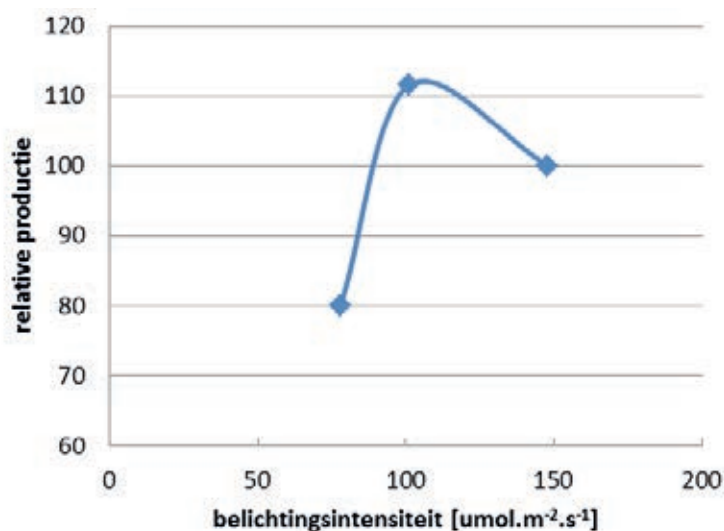
Figuur 9 Productieniveaus van roos 'Passion' van groepen telers geclassificeerd in drie belichtingsniveaus (Vermeulen and García 2009).
