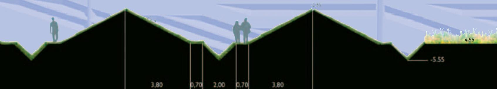
Het standaardprofiel van de ribbels voor Buitenschot.
