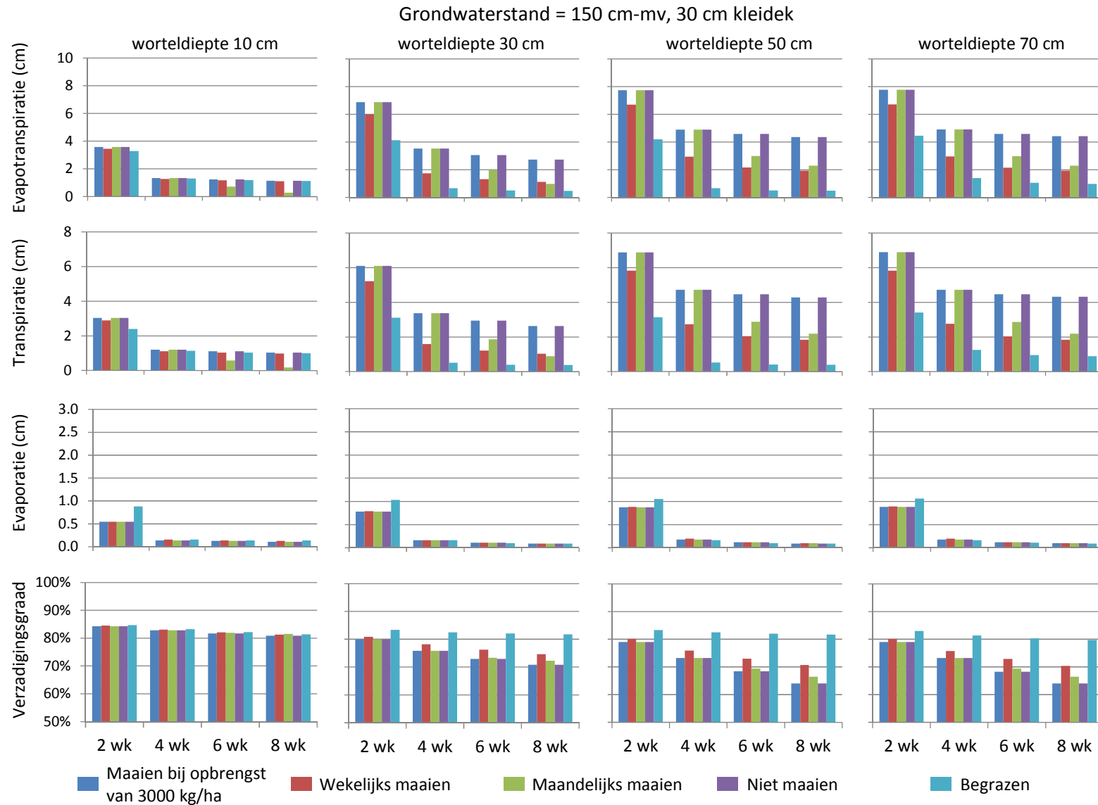
Bijlage 6. Twee wekelijkse verdampingstotalen en verzadigingsgraden van veendijken met 30 cm kleidek bij een grondwaterstand van 150 cm-mv vanaf 1 mei
