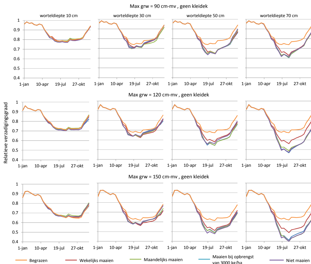
Figuur 5. Relatieve verzadigingsgraad van de bovenste meter van een veendijk zonder kleidek bij 3 verschillende grondwaterstanden en 4 verschillende worteldiepten gedurende het meteorologische jaar 1976
