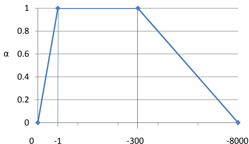
Figuur 1. Reductiefactor voor de gewasverdamping h in afhankelijkheid van de drukhoogte
