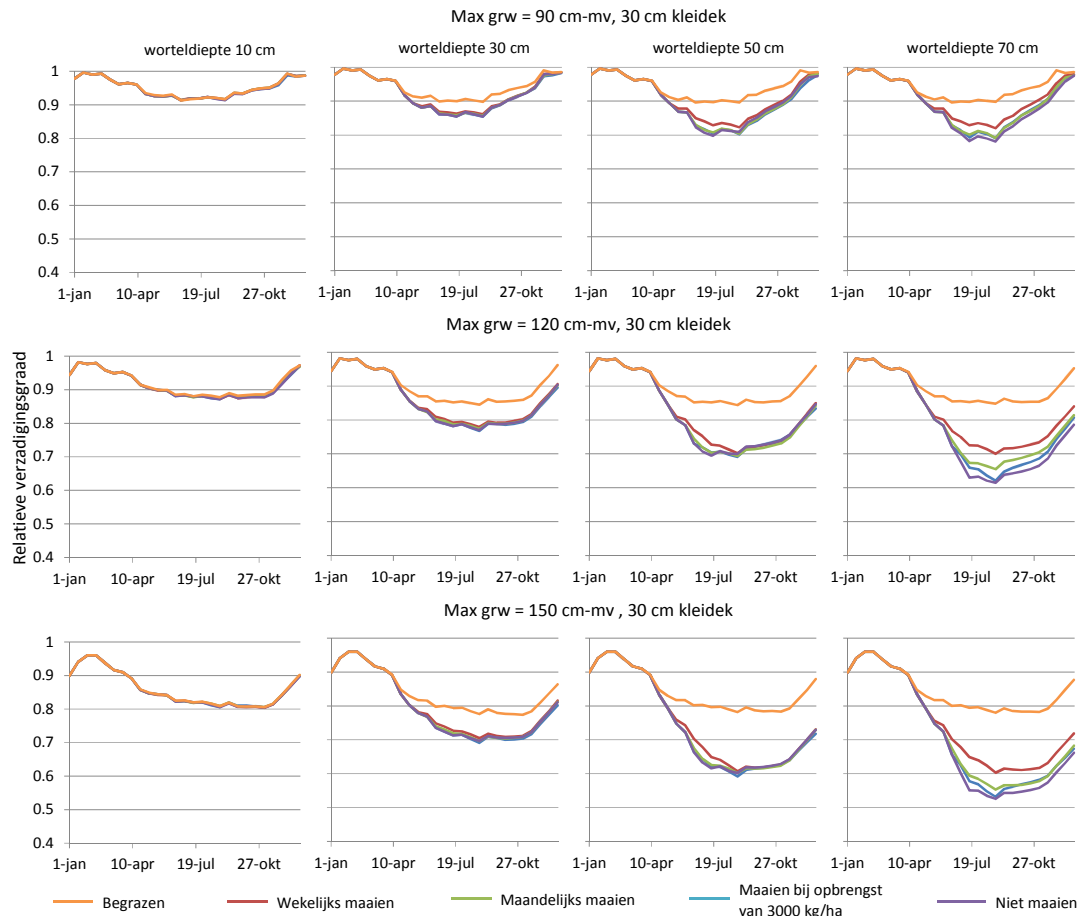
Figuur 6. Relatieve verzadigingsgraad van de bovenste meter van een veendijk met 30 cm kleidek bij 3 verschillende grondwaterstanden en 4 verschillende worteldiepten gedurende het meteorologische jaar 1976.
