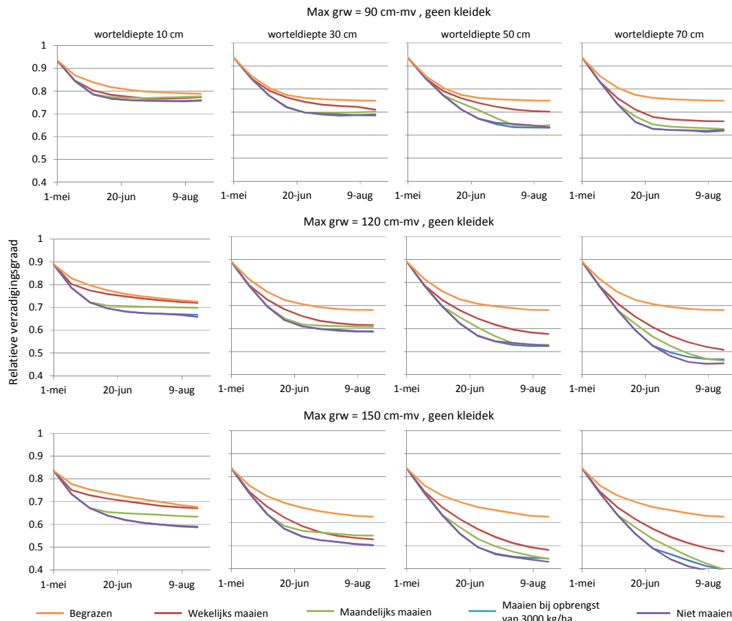
Figuur 3. Relatieve verzadigingsgraad van de bovenste meter van een uitdrogende veendijk zonder kleidek bij 3 verschillende grondwaterstanden en 4 verschillende worteldiepten gedurende de periode 1 mei tot 21 augustus.
