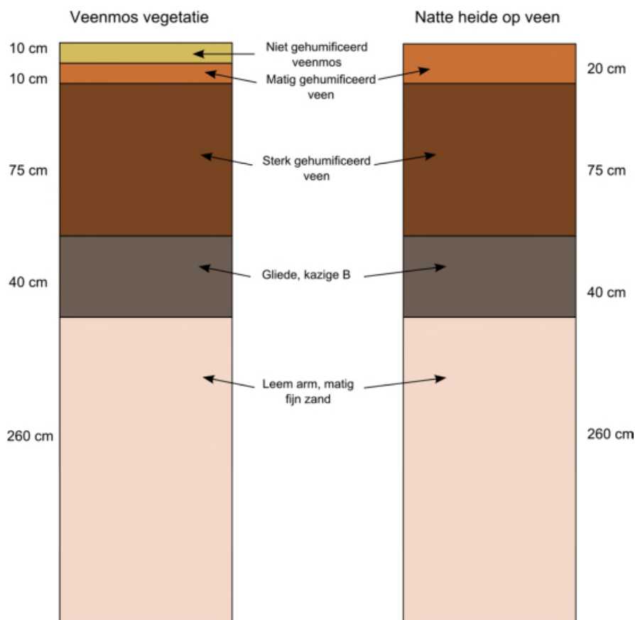
Figuur 2-1. Schematische weergave bodemopbouw in SWAP met (A) veenmos en (B) natte heide als top laag.
