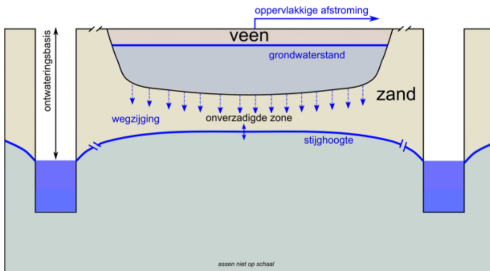
Figuur 1-2 Schematische weergave en definities van een schijnspiegelsysteem.
