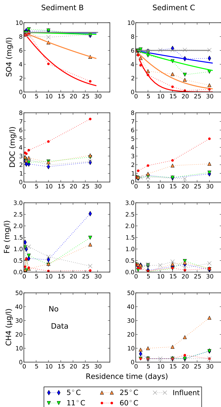
Figuur S-3: Analyseresultaten met toenemende verblijftijd. De punten en gestippelde lijnen geven de meetdata weer, voor \text{SO}_4 zijn tevens de resultaten weergegeven van \text{SO}_4 concentraties op basis van een Monod sulfaatreductie model (gesimuleerd met PHREEQC/PEST).
