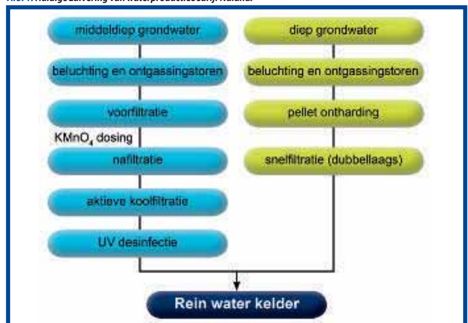
Afb. 1: Huidige zuivering van waterproductiebedrijf Nuland.
