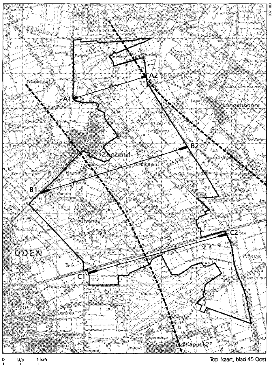
Fig. 2 Ligging van de geologische dwarsdoorsneden en breuken
