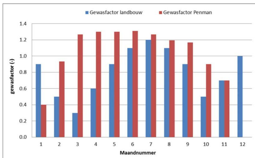
Figuur 3 Gewasfactoren voor de omrekening van de referentie gewasverdamping naar de potentiële verdamping van open water (Penman) en landbouwgewassen.
