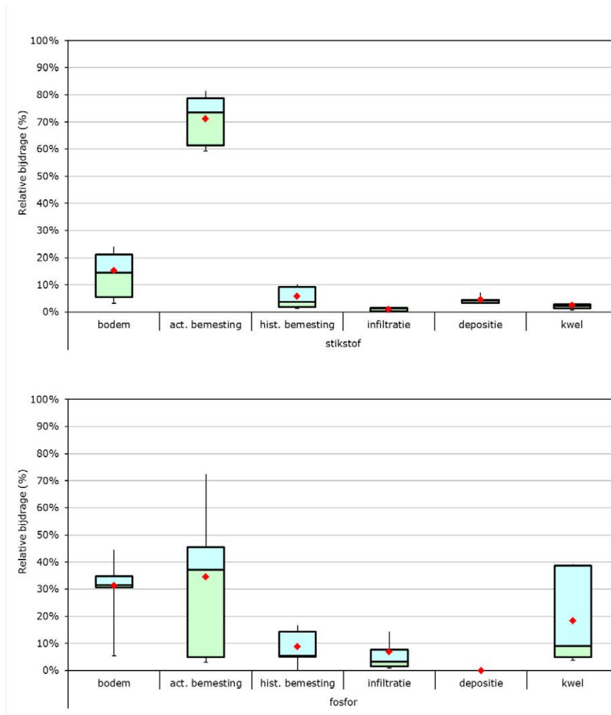
Figuur 9 Relatieve bijdrage van de verschillende nutriëntenbronnen aan de uit- en afspoeling vanuit landbouwgronden voor deelgebied Vier Noorderkoggen Hoog (boven stikstof, onder fosfor).
