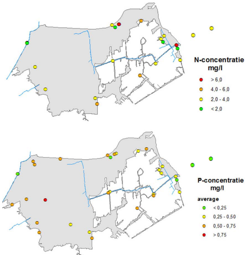
Figuur 7 Gemiddelde stikstof- en fosforconcentratie (mg/l) van meetpunten in en nabij deelgebied Vier Noorderkoggen Hoog voor de periode 2000-2009.
