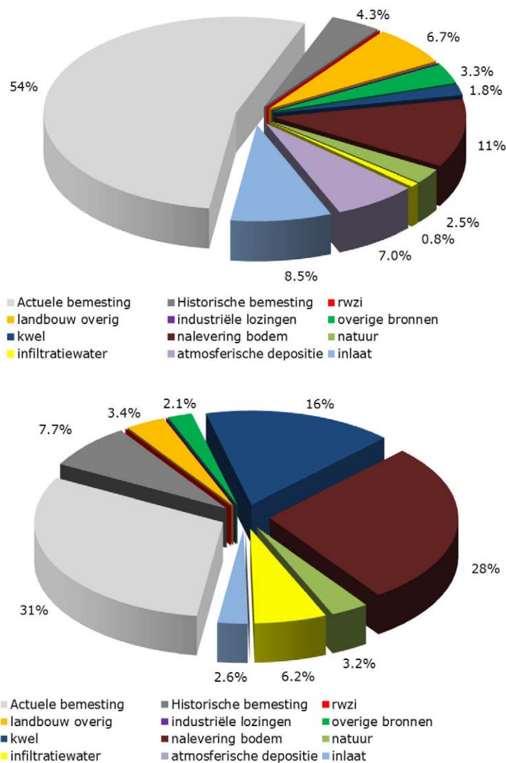
Figuur 10 Relatieve bijdrage van de verschillende nutriëntenbronnen aan de belasting van het oppervlaktewater voor deelgebied Vier Noorderkoggen Hoog (boven stikstof, onder fosfor), waarbij de uit- en afspoeling is onderverdeeld naar herkomst.
