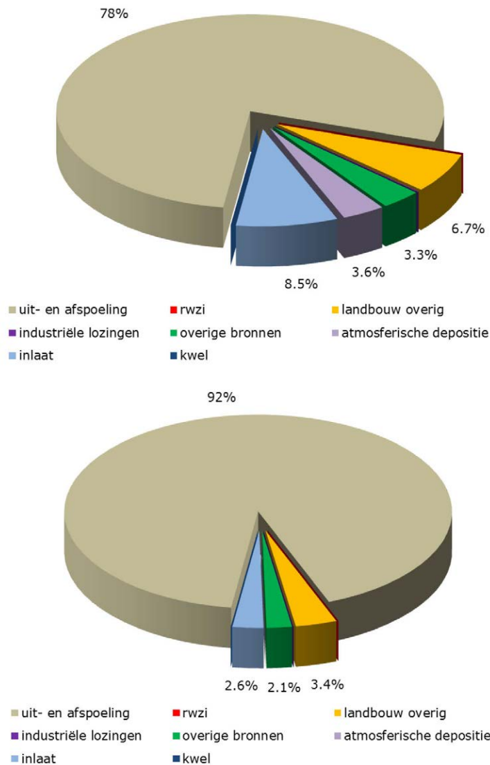
Figuur 8 Relatieve bijdrage van de verschillende nutriëntenbronnen aan de belasting van het oppervlaktewater voor deelgebied Vier Noorderkoggen Hoog (bovenste figuur stikstof, onderste figuur fosfor).
