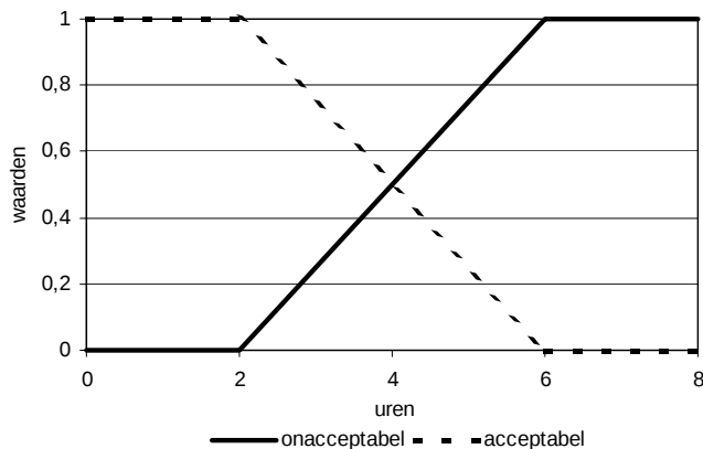
Figuur 17 Membershipfunctie van de blootstellingsduur. Figure 17 Membership function of the duration of exposure.
