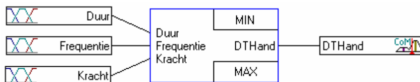
Figuur 21 Fuzzy-logicstructuur van beoordeling van een individuele duw/trek-handeling. Figure 21 Fuzzy logic structure of the assessment of one push/pull action.
