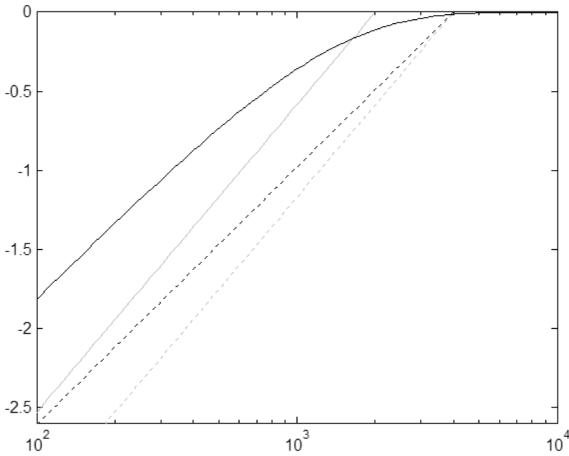
Afbeelding 11: Verlagingskegel(s) volgens De Vries (1974), maar voor een onttrekking van 6.5 miljoen m 3 /j. De getrokken lijn is voor de wintertoestand, de gestippelde voor de zomer. De grijze lijnen zijn die van het RID (1955).
