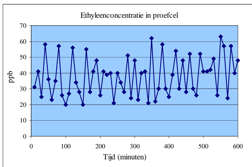
Figuur 1. Het principe van ethyleen-gestuurde ventilatie. Ethyleengehaltes in een proefcel met zure bollen. Ventilator aan bij waarden boven 50 à 60 ppb, ventilator uit bij waarden boven 20 à 30 ppb.
