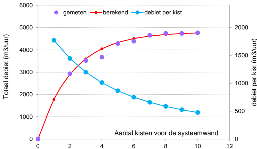
Figuur 3: Totaal debiet laag 2 vs aantal kisten.
