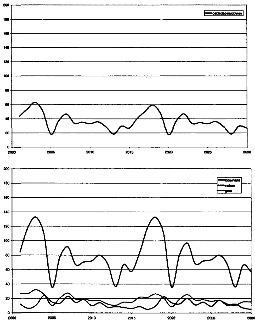
De gebiedsgemiddelde nitraatconcentratie en de nitraatconcentratie per bodemgebruik ( \text{mg.l}^{-1} \text{NO}_3 ) in het bovenste grondwater in de periode 2000-2030 voor de huidige situatie.
