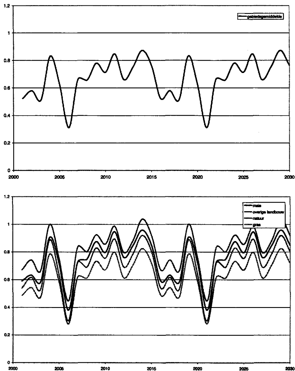
Tijdverloop van de gebiedsgemiddelde afvoer en de afvoer per bodemgebruik ( m^3 \cdot ha^{-1} ) in de periode 2000-2030 voor de huidige situatie .
