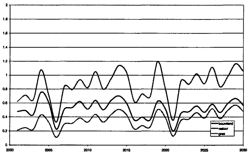
Tijdverloop van de gebiedsgemiddelde fosforvracht en de vracht per bodemgebruik ( \text{kg} \cdot \text{ha}^{-1} \text{P} ) naar het oppervlaktewater in de periode 2000-2030 voor de plansituatie.
