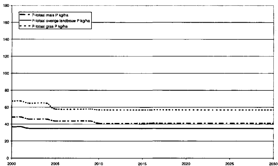
Figuur 10 Aanvoer van fosfor ( \text{kg} \cdot \text{ha}^{-1} \text{P} ) via bemesting op grasland, mais en overige landbouw in de periode 2001-2030
