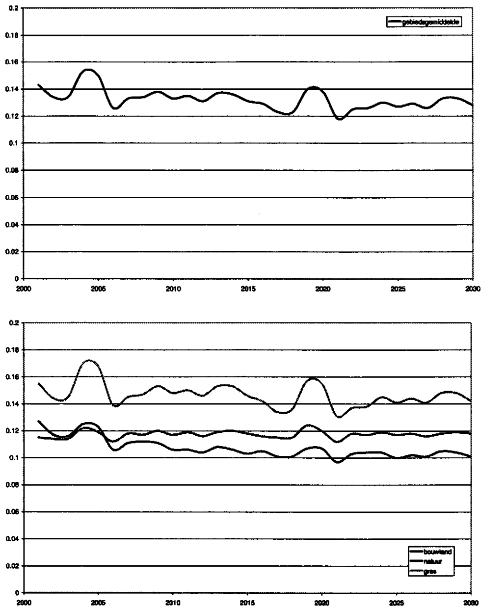
Tijdverloop van de gebiedsgemiddelde fosforconcentratie en de concentratie per bodemgebruik (mg.l -1 P) in de afvoer naar het oppervlaktewater in de periode 2000-2030 voor de huidige situatie.
