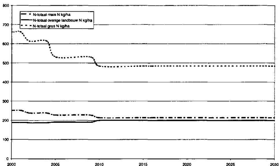
Figuur 9 Aanvoer van stikstof ( \text{kg} \cdot \text{ha}^{-1} \text{ N} ) via bemesting op grasland, maïs en overige landbouw in de periode 2001-2030
