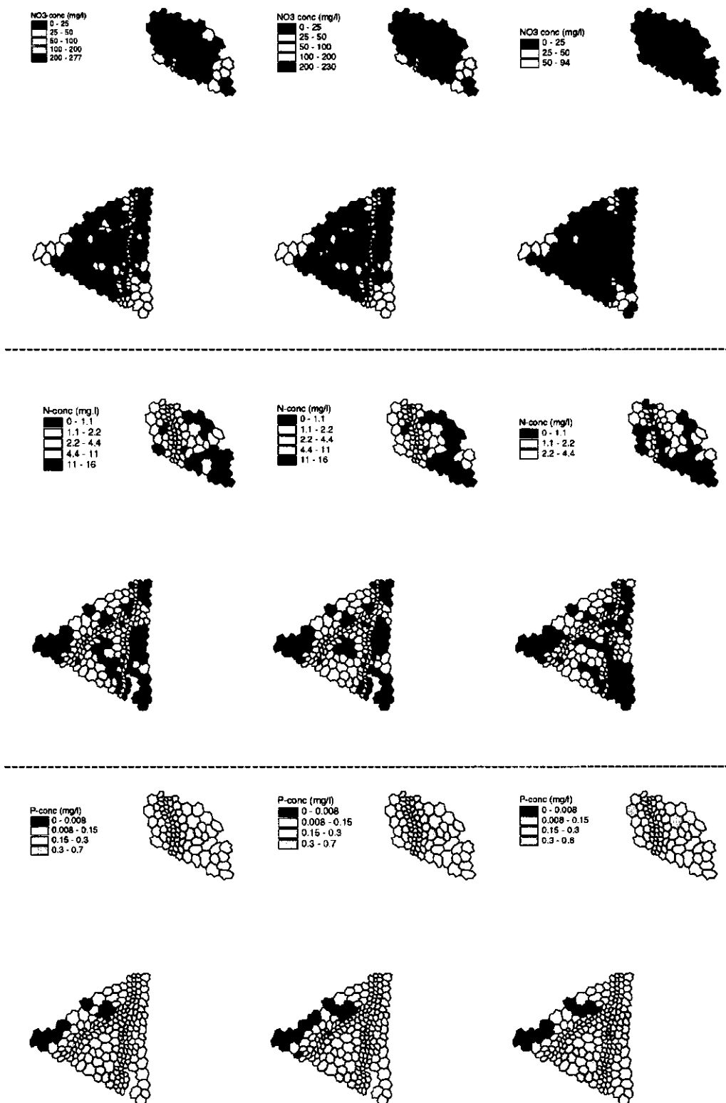
Figuur 11 Berekende nitraat-, stikstof- en fosforconcentraties in 2000 (links), in 2030 voor de huidige situatie (midden) en in 2030 voor de plansituatie (rechts).
