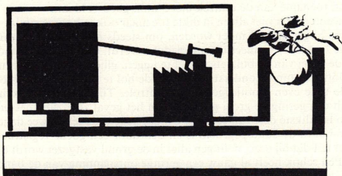
FIG. 9. Groeimeter volgens STENZ (28).
