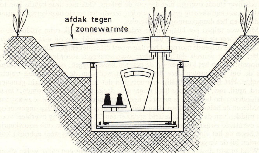
FIG. 13. Schema van de ingebouwde balans.
