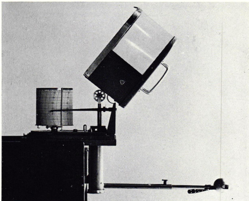
FOTO 4. Verbeterde groeimeter, geconstrueerd door het K.N.M.I., waarbij van de oorspronkelijke werd uitgegaan. PHOTO 4. Improved growth graph.
