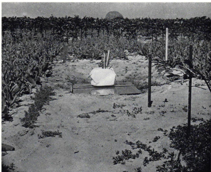
FOTO 13. Ingebouwde balans, overzicht, zonder afdak tegen de zonnewarmte. PHOTO 13. Built-in balance, general view, without screen against insolation.
