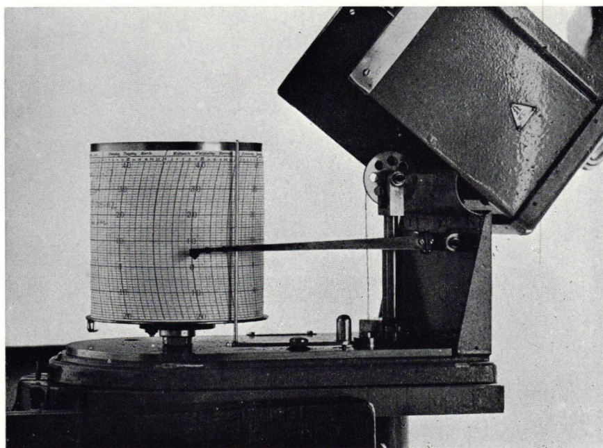
FOTO 5. Dezelfde groeimeter als op foto 4. PHOTO 5. The same growth graph as shown on photo 4.
