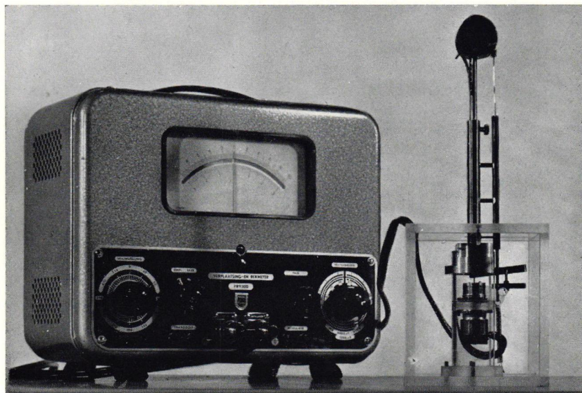
FOTO 15. Groeimeter, rechts, gebaseerd op een verplaatsingsopnemer (24), onderin, met de bijbehorende meetbrug.
