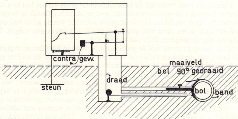
FIG. 8. Schema van de groeimeter.
