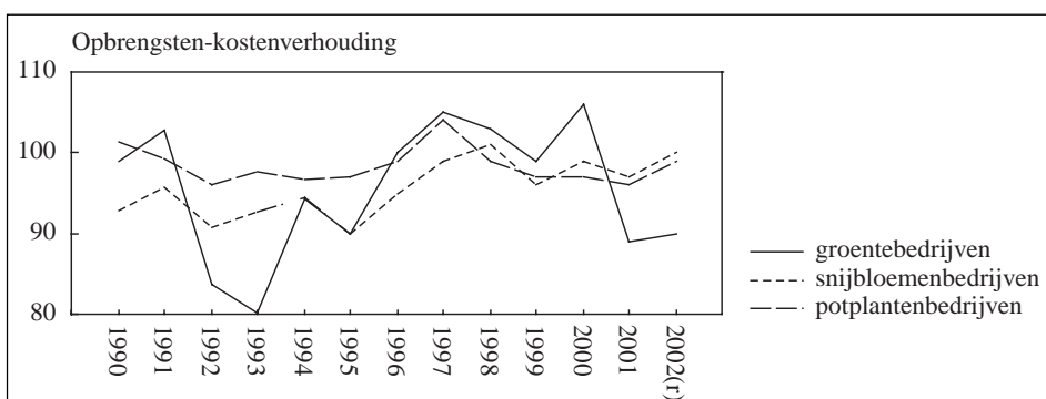
Figuur 1 Ontwikkeling opbrengst per 100 euro kosten op glastuinbouwbedrijven 1990-2002
