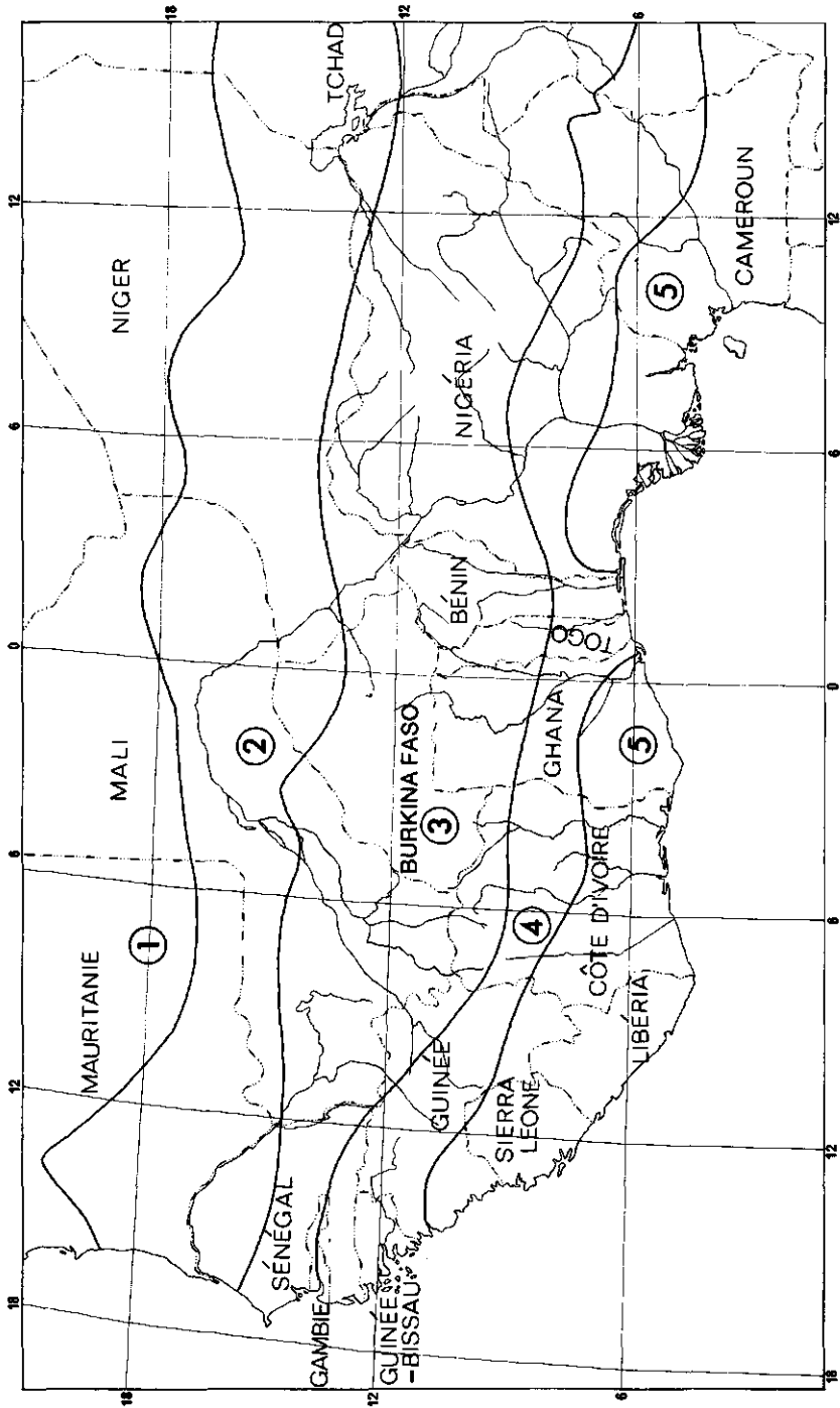
Carte des zones écologiques: 1. Sahara 2. Sahel 3. savanes soudanaises 4. savanes guinéennes 5. forêt.
