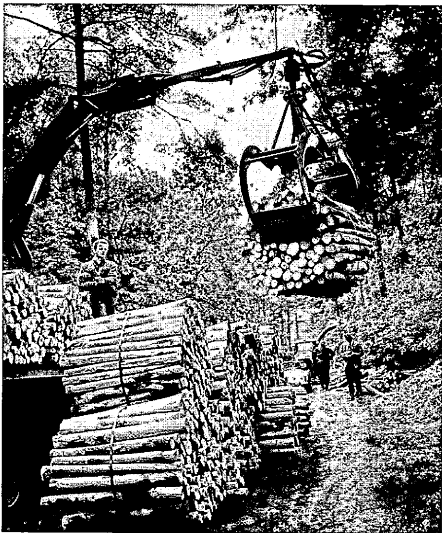
Laden van gebundeld sortiment met een over het laadplatform verplaatsbare hydraulische kraan.
