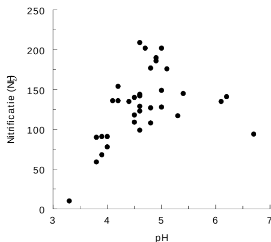
Figuur 4.11: pH-optimum voor potentiële nitrificatie.
