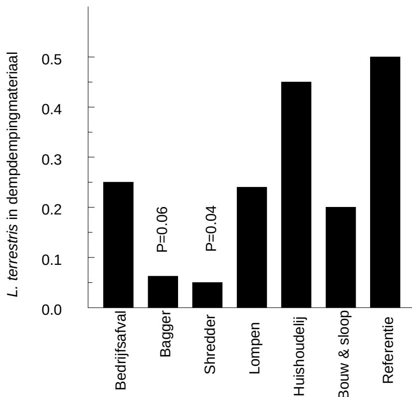
Figuur 4.12: Het deel van de kolommen waarin regenwormen zich in het dempingmateriaal bevonden aan het einde van de bioturbatieproef.
