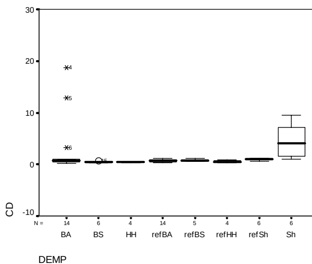
Figuur 7.1: Boxplot van de beschikbare gehalten cadmium in de deklaag boven de verschillende dempingcategorieën en de hierbij horende referenties.
