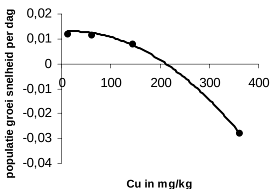
Figuur 7.4: Populatie groeisnelheid van L. rubellus onder invloed van koper, waarbij de onderhoudskosten zijn verhoogd (naar Klok & de Roos (1996). De gefitte lijn (-3.87 \cdot 10^{-7} Cu^2 + 3.11 \cdot 10^{-5} Cu + 0.0115, R^2 \text{ ad } 0.999, F=0.015)
