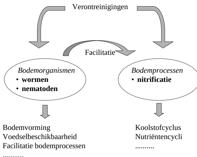
Figuur 5.1. Schematische weergave van relaties tussen verontreinigingen, bodemorganismen en bodemprocessen. Vetgedrukt staan de parameters weergegeven die in het huidige verificatieonderzoek bestudeerd zijn.
