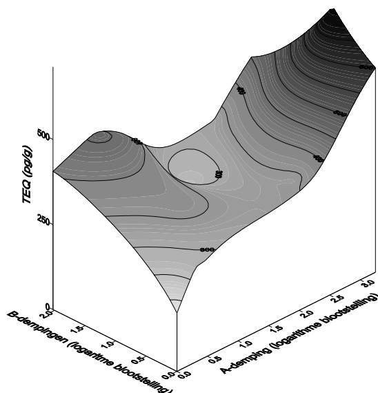
Figuur 8.3. Relatie tussen blootstelling aan A-dempingen en B-dempingen (volgens D2) enerzijds en TEQ waarden in kuikens uit eieren van grutto's en Kievieten anderzijds, gebaseerd op geïnterpoleerde data (kriging).
