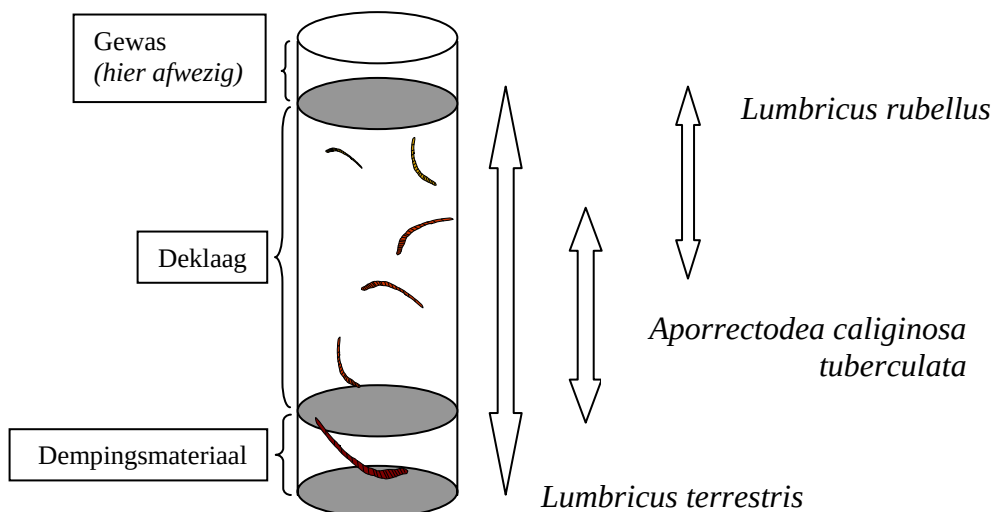
Figuur 4.13. Schematisch transport van stoffen (pijlen) tussen dempingsmateriaal en deklaag door verschillende regenwormen in de bioturbatieproef.
