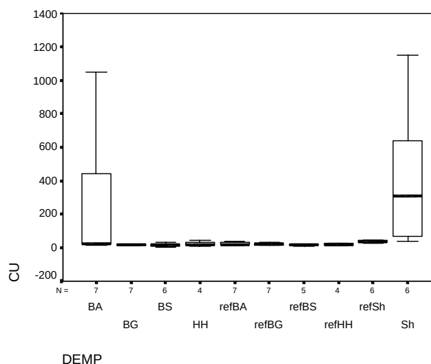
Figuur 7.2: Boxplot van de beschikbare gehalten koper in de deklaag boven de verschillende dempingcategorieën en de hierbij horende referenties.
