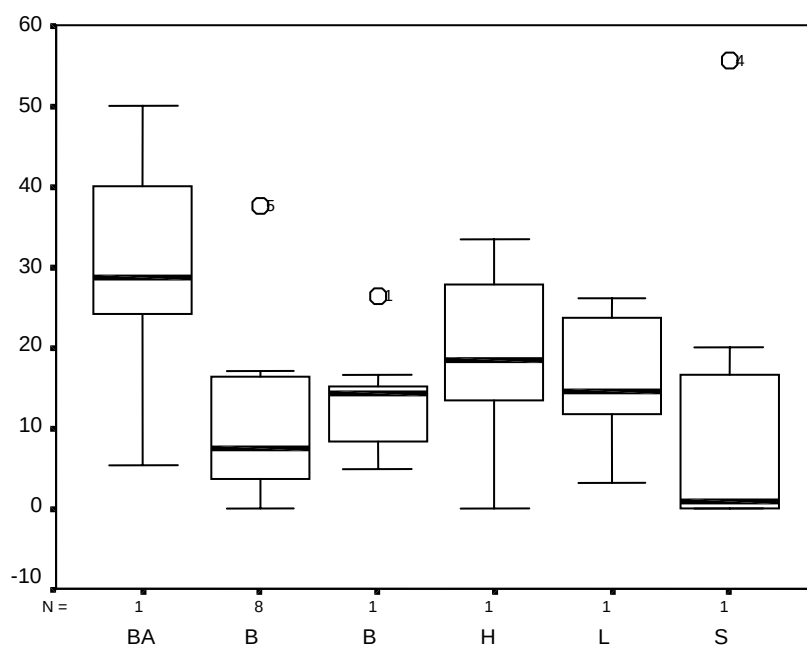
Figuur 3.4: Boxplot van het percentage sub-adulten L. rubellus op de verschillende dempingcategorieën onder de aanname dat de referenties gelijk zijn aan de deklagen boven de demping.
