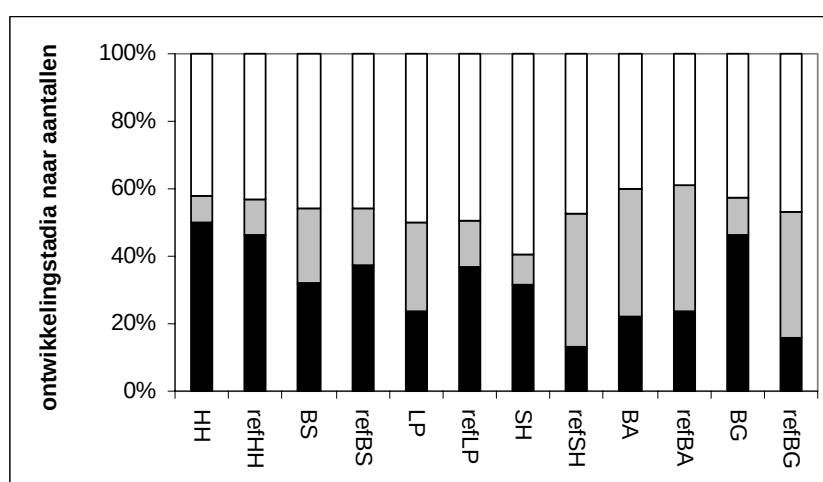
Figuur 4.3. Populatieopbouw in adulten (zwart), sub-adulten (grijs) en juvenielen (wit) van L. rubellus naar aantallen op de verschillende dempingmateriaal en bijborende referenties.
