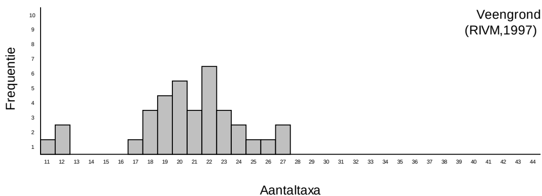
Figuur A7.1. Frequentieverdelingen van aantallen taxa nematoden in deklagen (DEK) en referentiegrasland (REF) in de Krimpenerwaard en in landelijke referenties (Landelijk Meetnet Bodemkwaliteit, RIVM) voor veenweidegrond.
