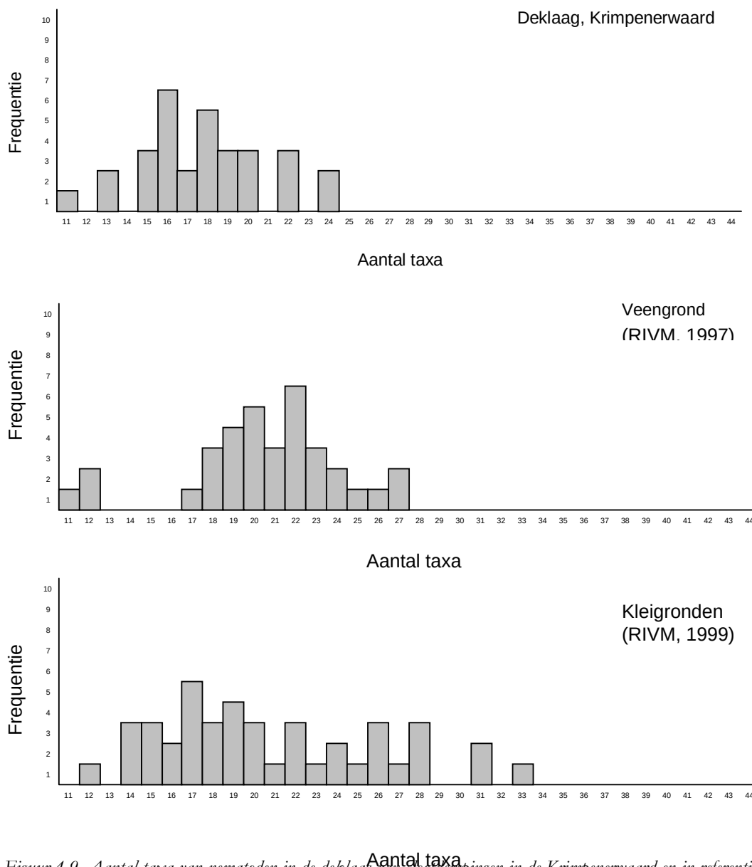
Figuur 4.9. Aantal taxa van nematoden in de deklaag van slootdempingen in de Krimpenerwaard en in referentie klei- en veengronden.
