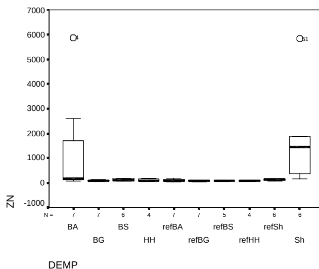
Figuur 7.3: Boxplot van de beschikbare gehalten zink in de deklaag boven de verschillende dempingcategorieën en de hierbij horende referenties.
