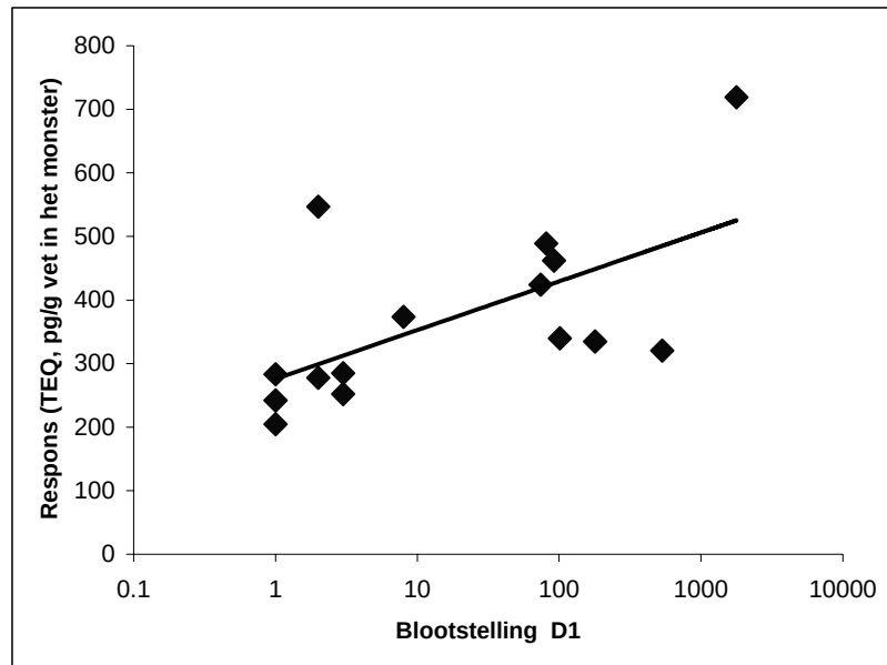
Figuur 1. Verontreiniging in weidevogeleieren (TEQ-response uitgedrukt als pg/g TCDD in het vet van de monsters) als functie van blootstelling aan verdachte slootdempingen ongeacht de afdekking, in de Krimpenerwaard binnen een straal van 300m rond het nest.
