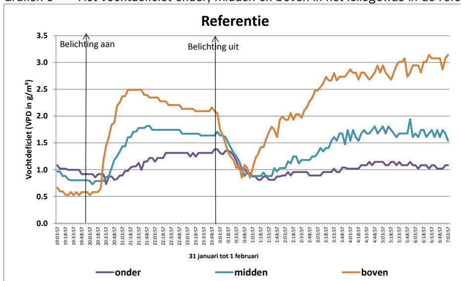
Grafiek 6 Het vochtdeficiet onder, midden en boven in het leliegewas en in het pad en de stand van de ventilator in HNT in de nacht van 31 jan op 01-02
