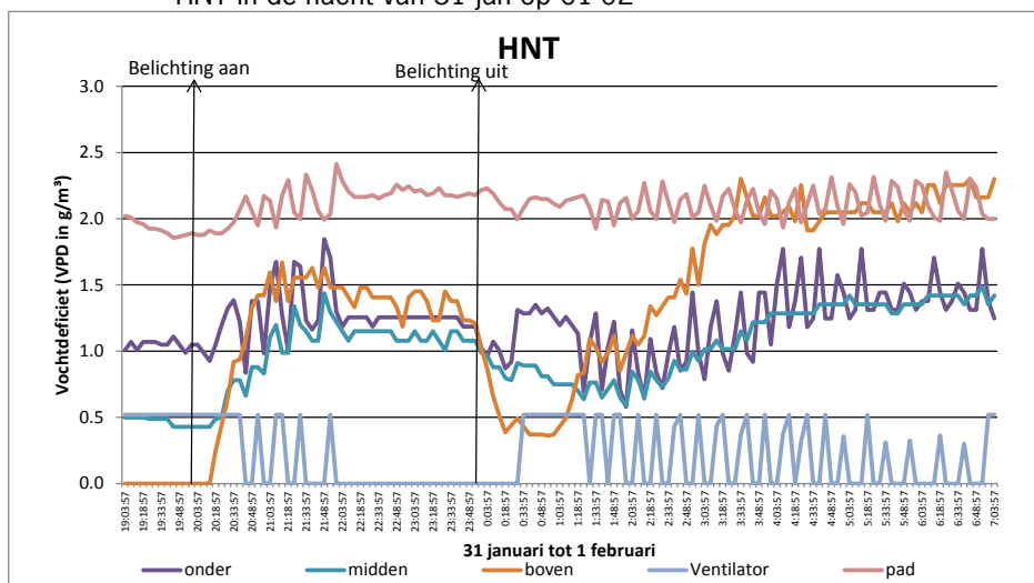
Grafiek 6 Het vochtdeficiet onder, midden en boven in het leliegewas en in het pad en de stand van de ventilator in HNT in de nacht van 31 jan op 01-02
