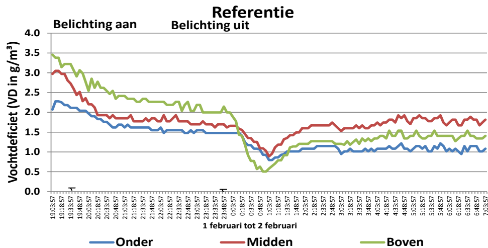
Grafiek 10 Het vochtdeficiet onder, midden en boven in het leliegwas in HNT in de nacht van 01-02 op 02-02
