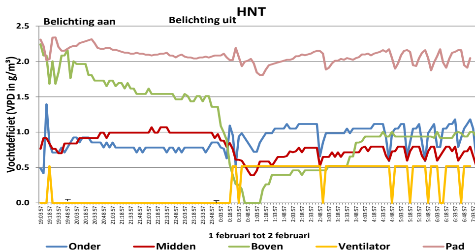
Grafiek 10 Het vochtdeficiet onder, midden en boven in het leliegwas in HNT in de nacht van 01-02 op 02-02
