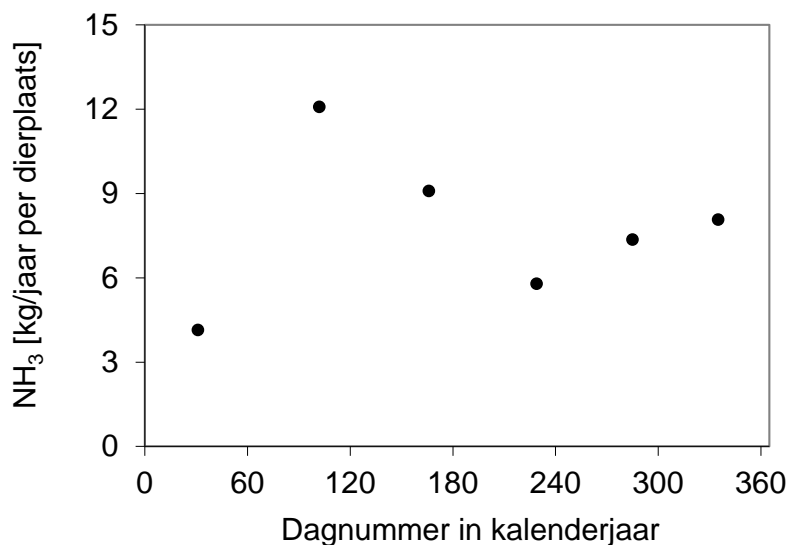
Figuur 5 Gemiddelde NH 3 -emissie op alle verschillende meetdagen
