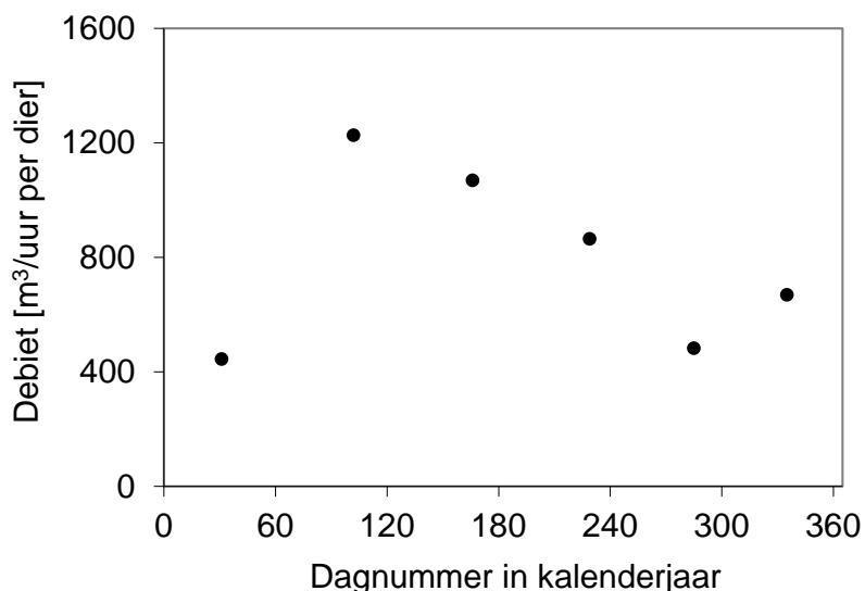
Figuur 4 Gemiddelde ventilatie-debiet [m 3 /uur per dier] op alle verschillende meetdagen
