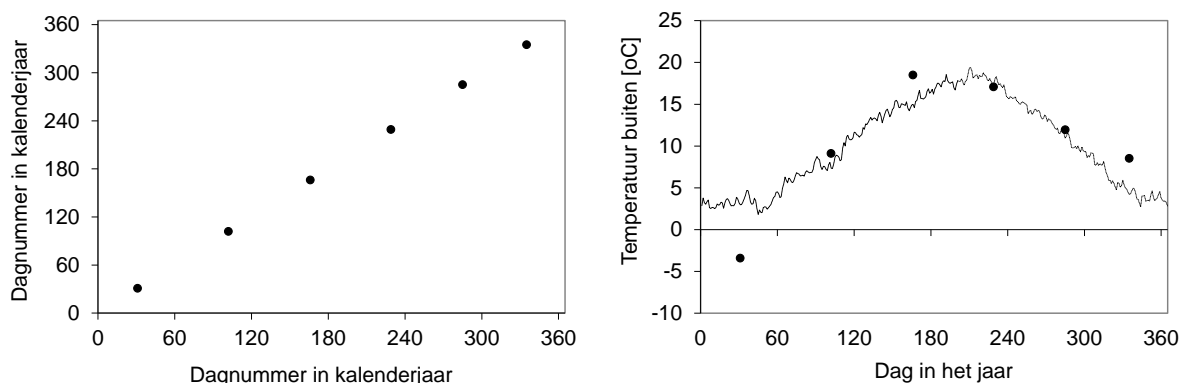
Figuur 3 Verdeling van de metingen over het jaar (a), en de buitentemperatuur (b) vergeleken met de gemiddelde waarden gemeten over de jaren 1991-2010 bij het KNMI-weerstation Stavoren ( www.knmi.nl ; als stippellijn weergegeven).
