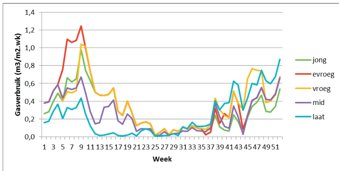
Figuur 1. Berekend gasverbruik ( \text{m}^3/\text{m}^2.\text{wk} ) voor de vijf verschillende teeltafdelingen indien er geen vochtregeling wordt aangehouden.
