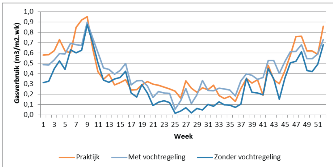
Figuur 4. Gasverbruik ( \text{m}^3/\text{m}^2.\text{wk} ) gemiddeld bij praktijkbedrijven, en volgens de berekeningen zonder vochtregeling en met vochtregeling (streefwaarde 85% RV).
