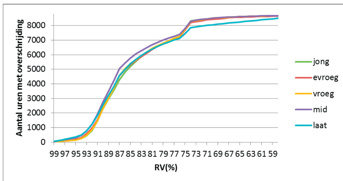
Figuur 2. Jaarduirkromme; het aantal uren is dat een bepaalde RV is overschreden is uitgezet tegen de RV.
