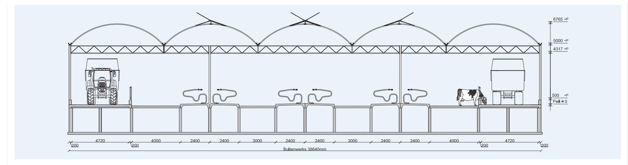
↓ DOORSNEDE SERRESTAL 0+6+0.
