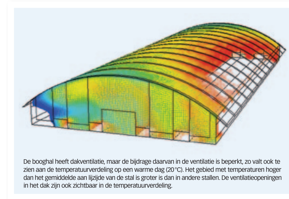
VENTILATIEPLAATJE BOOGSTAL.
