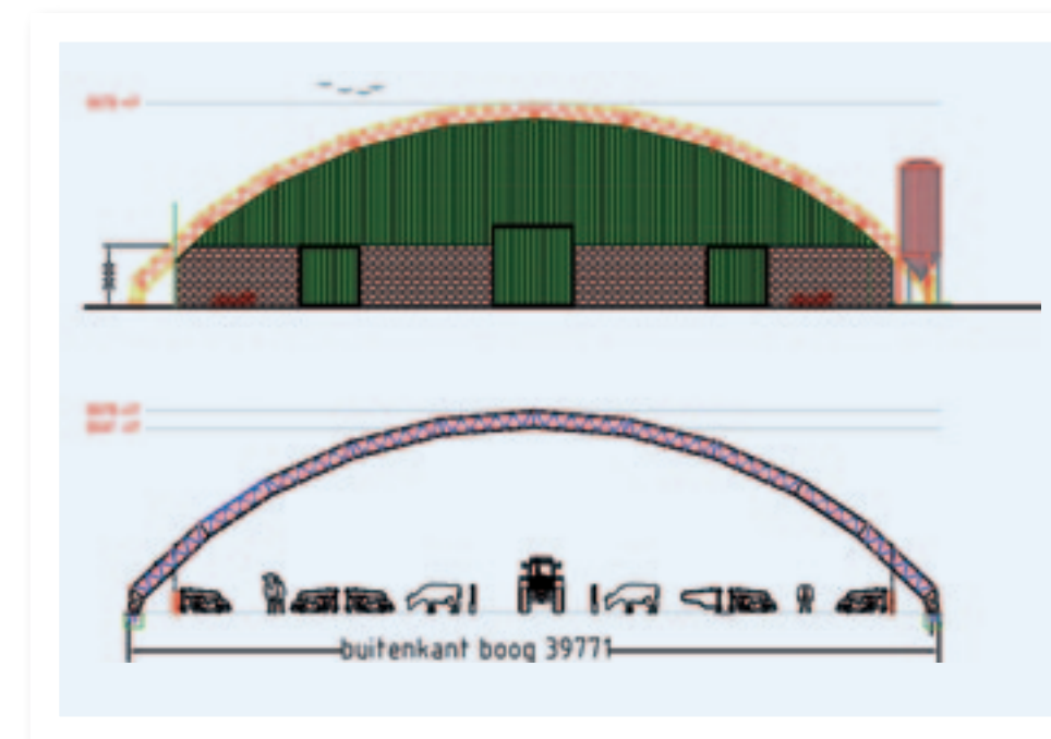
↑ DOORSNEDE BOOGSTAL 3+3.
