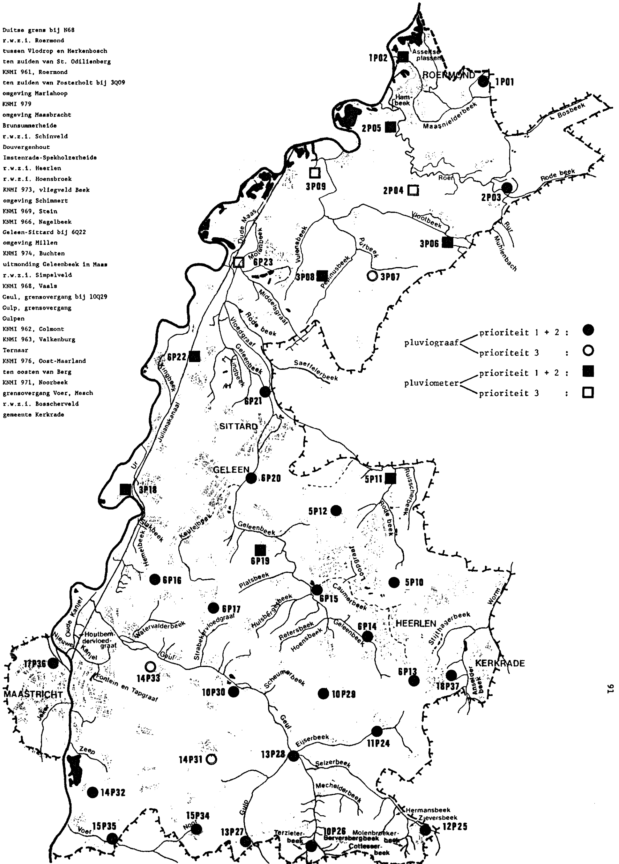
Figuur 31 Gewenste lokatie voor de neerslagmeetpunten.
