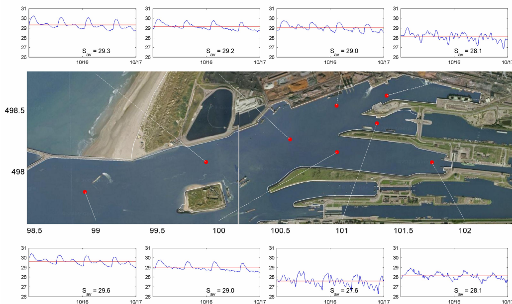
Figuur 4.4 Gemodelleerde zoutgehalten nabij de bodem gedurende 4 getijcycli
