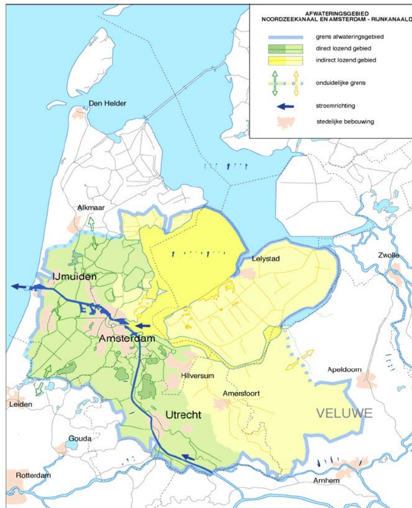
Figuur 3.3 Afwateringsgebied Noordzeekanaal en Amsterdam-Rijnkanaal (uit: Akkermans, 2003)
