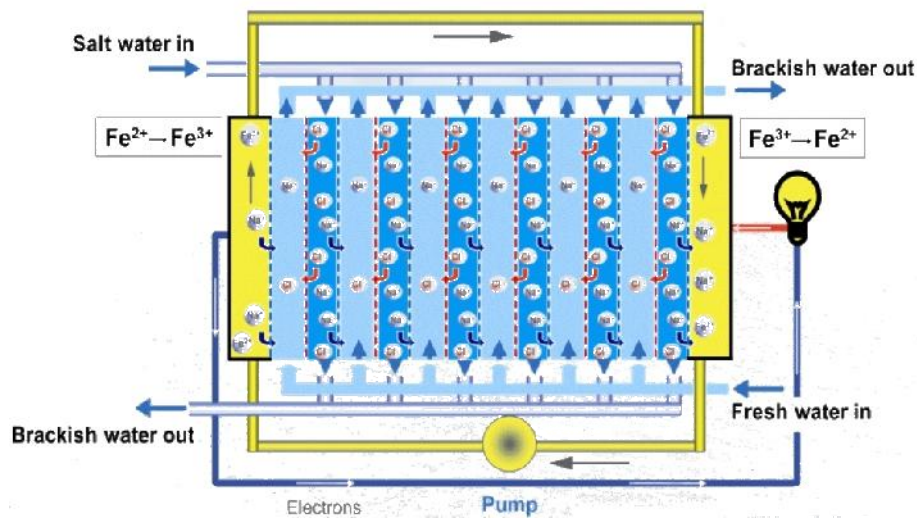
Figuur 2.2 Schematische weergave van een RED installatie, uit Molenbroek (2007), origineel: presentatie REDSTACK
