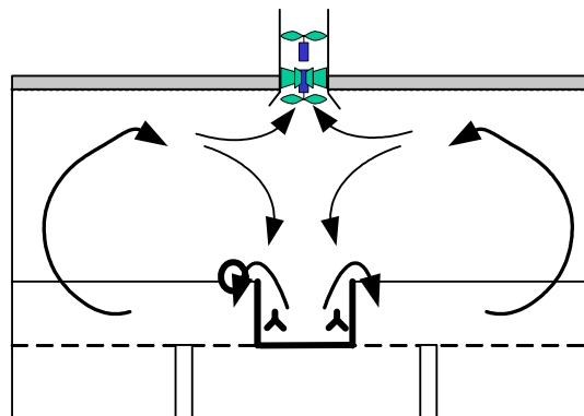
Dwarsdoorsnede afdeling
