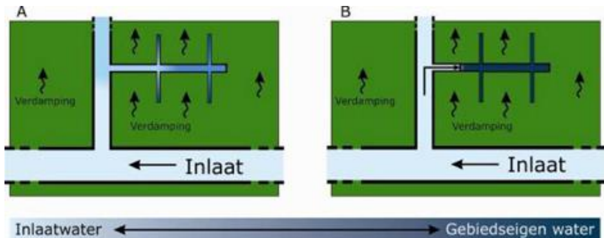
Figuur 4. De verspreiding van inlaatwater in droge perioden met veel verdamping. (A): denkmodel vroeger: inlaatwater mengt met gebiedseigen water en dringt helemaal door tot in de 'haarvaten van het oppervlaktewatersysteem'; (B): huidig denkmodel: minder menging, inlaatwater 'duwt' gebiedseigen water terug de haarvaten in. Bron: Siderius e.a. 2011
