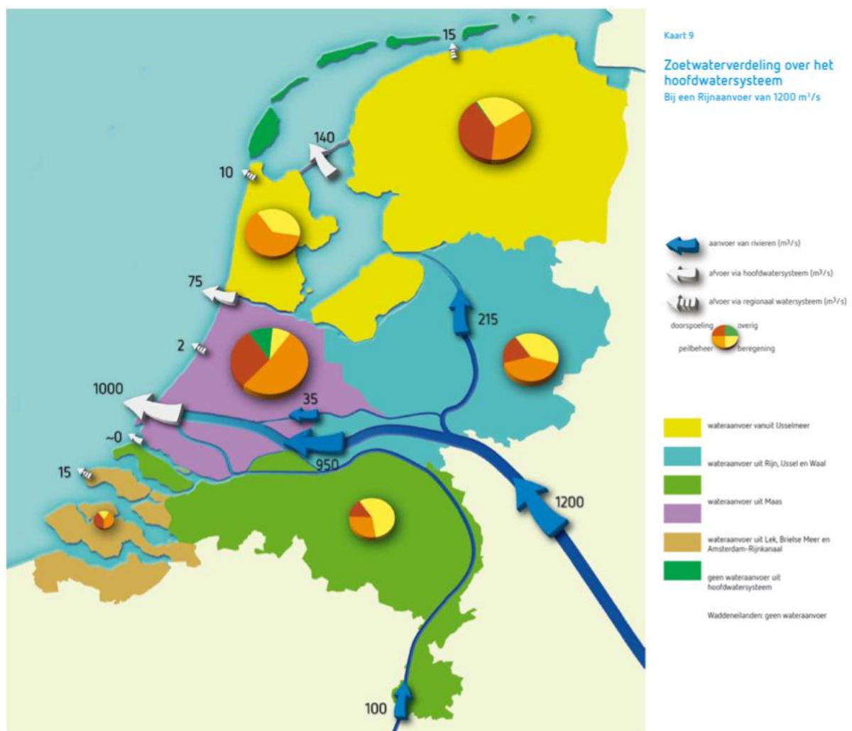
Figuur 1. Zoetwaterverdeling en aanvoer vanuit het hoofdwatersysteem bij Rijnaanvoer van 1200m 3 /s-1 (vergelijk: zomergemiddelde afvoer 1976 ( 1115 m 3 /s en 1967 (2250 m 3 /s) Bron: Nationaal Waterplan 2009-2015. N.B. De hier gepresenteerde getallen en verdeling wijken af van de resultaten uit latere studies, o.a. Witteveen en Bos (2011), Klijn et al. (2012)
