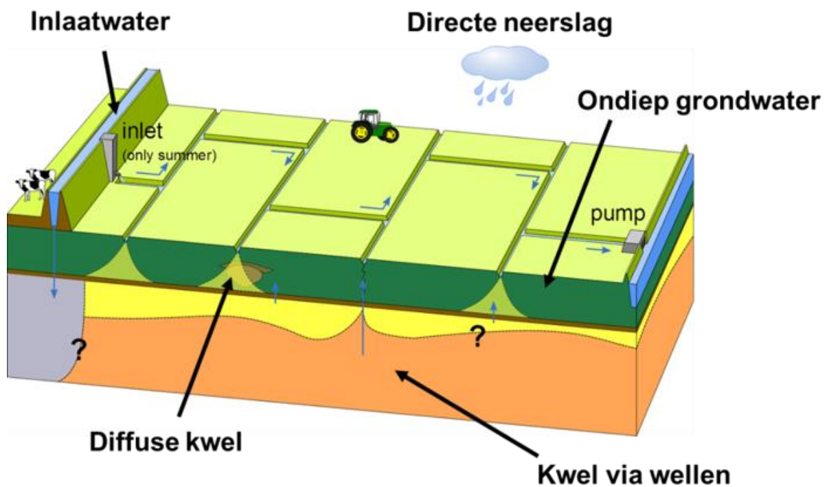
Figuur 3. Overzicht van soorten (bronnen van) water die in een diepe polder in de sloot mengen.
