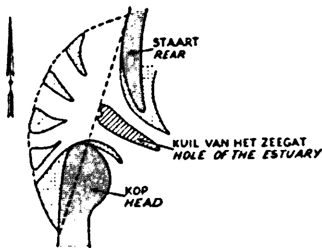
AFB. 54. Principe van de vorming van strandwallen aan weerszijden van een zeevat onder invloed van een langs de kust staande stroming (volgens VAN VEEN).
