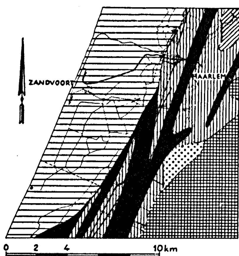
AFB. 48. Geologische gesteldheid in de omgeving van Bennebroek.
