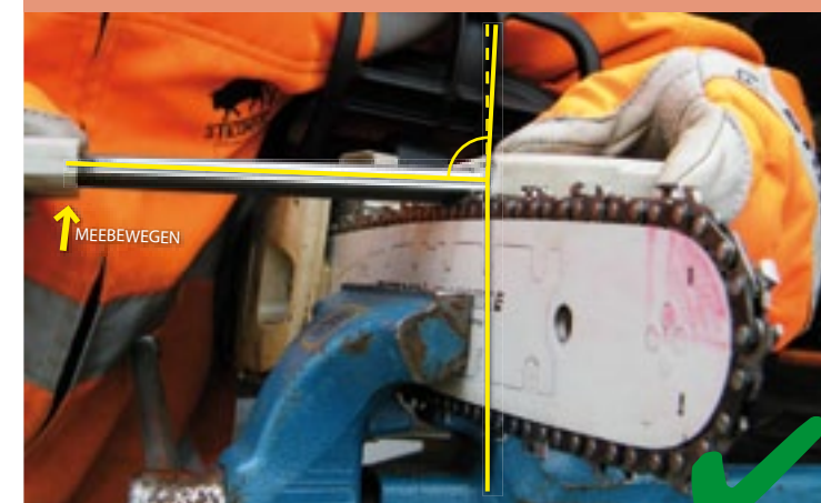
3 Meebewegen – Haaks, 90°, op de KETTING Door het rechterhandvat (op de foto links) iets op te tillen, beweegt u met de speling mee. De combivijlhouder blijft vlak over het dak van de beitel gaan. De vijl holt de punt op de juiste diepte uit. Bij deze Picco-ketting snijhoek B 75°.
