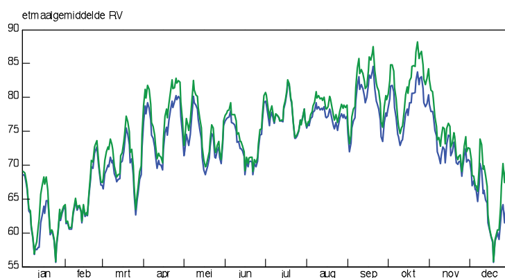
Figuur 17. Verloop etmaalgemiddelde RV in referentieteeelt (blauw) en in een teelt waarbij een hogere RV wordt toegelaten (groen), en die tot een besparing van 2 m 3 /m 2 aardgas per jaar leidt.
