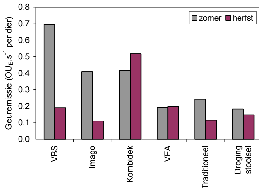
Figuur 5 Geuremissies tijdens meetperioden in de zomer en herfst van verschillende stalsystemen voor vleeskuikens (Scheer et al, 2003; Ogink en Lens, 2001).
