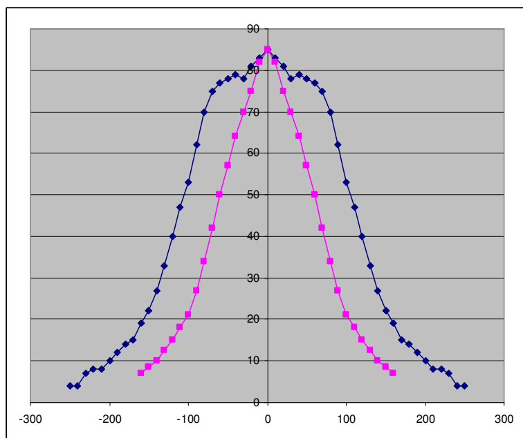
Figuur 9: Lichtverdeling van enkele lamp met verstrooiing folie.
