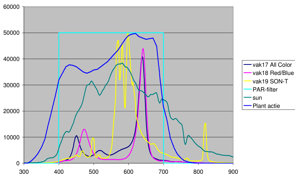
Figuur 33 : Gerealiseerd spectrum licht
