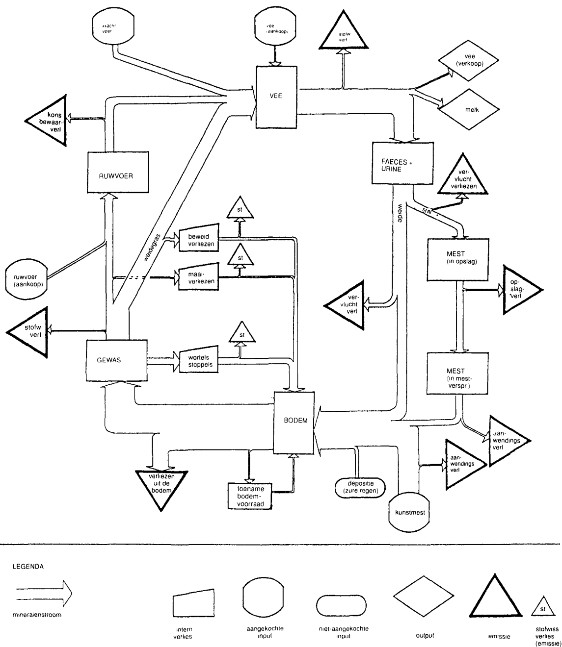
Figuur 1: Stikstofstromen op het rundveehouderijbedrijf (CLM, PR, CABO, 1988).
