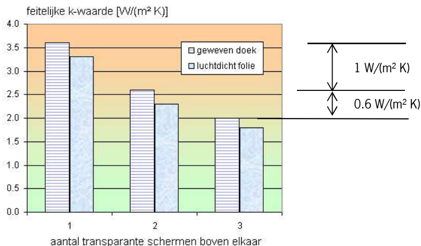
Figuur 9. Invloed van het aantal scherm lagen op de feitelijke k-waarde van een kas (met feitelijke k-waarde wordt het verwarmingsvermogen voor de overbrugging van het temperatuurverschil tussen binnen en buiten en is dus exclusief het warmteverbruik voor de verdamping). Voor de geweven doeken is een lek van 3 m 3 /(m 2 uur) verondersteld.
