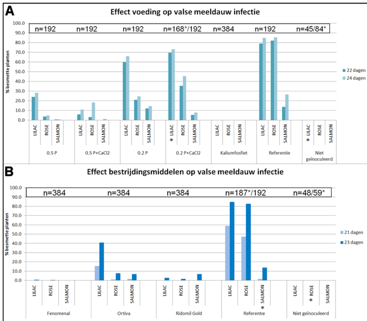
Figuur 5.3: (A) Effect van meststoffen en een plantversterker met kaliumfosfiet op valse meeldauw infectie 21 en 23 dagen na inoculatie. P^+ = 0,5 mmol P, en P^- = 0,2 mmol P. (B) Effect van gewasbeschermingsmiddelen op valse meeldauw infectie 21 en 23 dagen na inoculatie.
