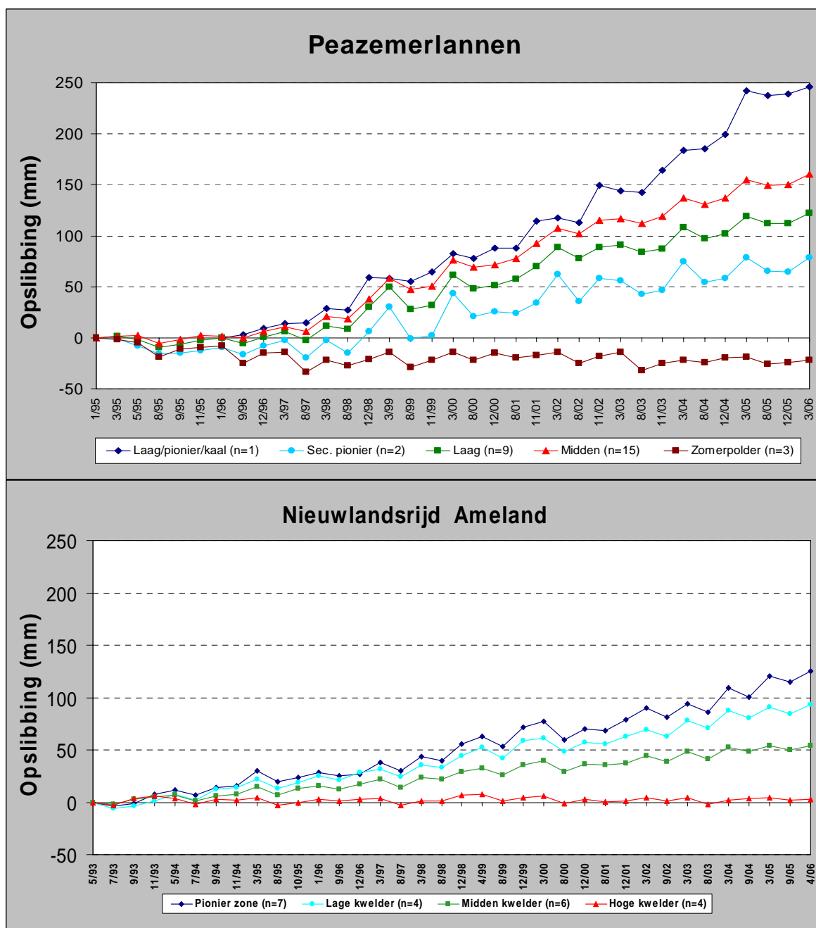
Figuur 5.3. Sedimentatie-erosie (SEB) metingen in de Peazemerlannen en op Ameland.
