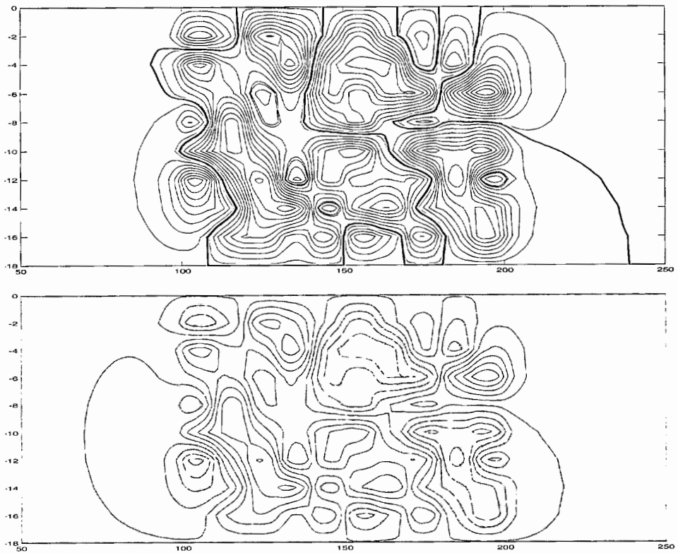
Figuur 8: Verschillende afbeeldingen van hetzelfde wervelpatroon, berekend met de stroomfunctie. In de bovenste figuur is de nulwaarde met een dikkere lijn aangegeven: dit geeft de grens aan tussen de linksom en rechtsom draaiende wervels. In de onderste figuur zijn de rechtsom draaiende wervels licht gekleurd en linksom draaiende wervels donker.
