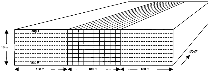
Figuur 1: Een gelaagd pakket spanningwater met een heterogeen-anisotrope zone in het midden.
