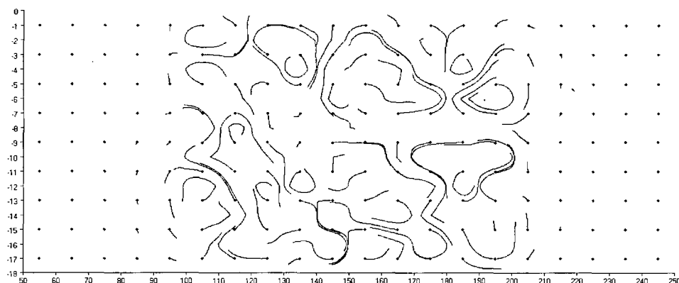
Figuur 2: Dwarsprofiel met 9 \times 20 geprojecteerde stroomlijnen berekend met MicroFEM. Om de stromingsrichting aan te geven beginnen alle stroomlijnen met een stip.
