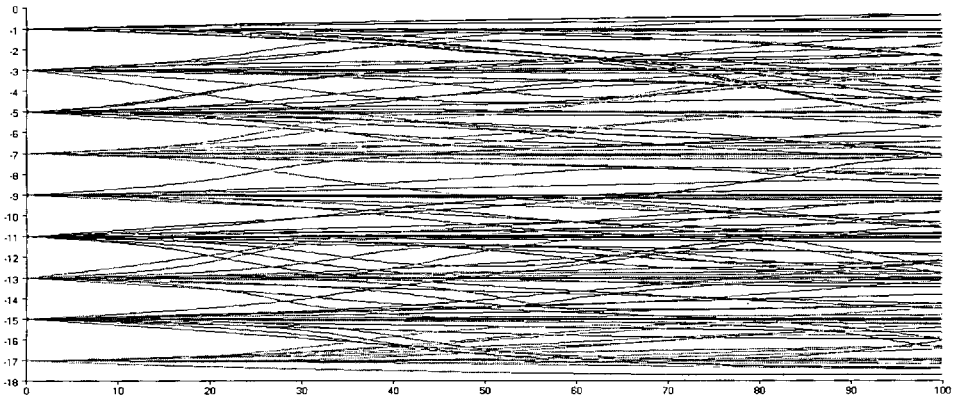
Figuur 3: Zuid-noord profiel met alle 9 * 20 stroomlijnen uit figuur 2 in zij aanzicht.
