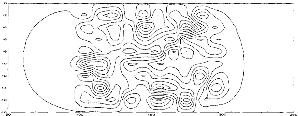
Figuur 9: Dwarsdoorsnede met rechtsom (licht gekleurd) en linksom (donker gekleurd) draaiende wervels in een model waarbij 45 graden is opgeteld bij de in tabel 1 gegeven anisotropierichtingen.
