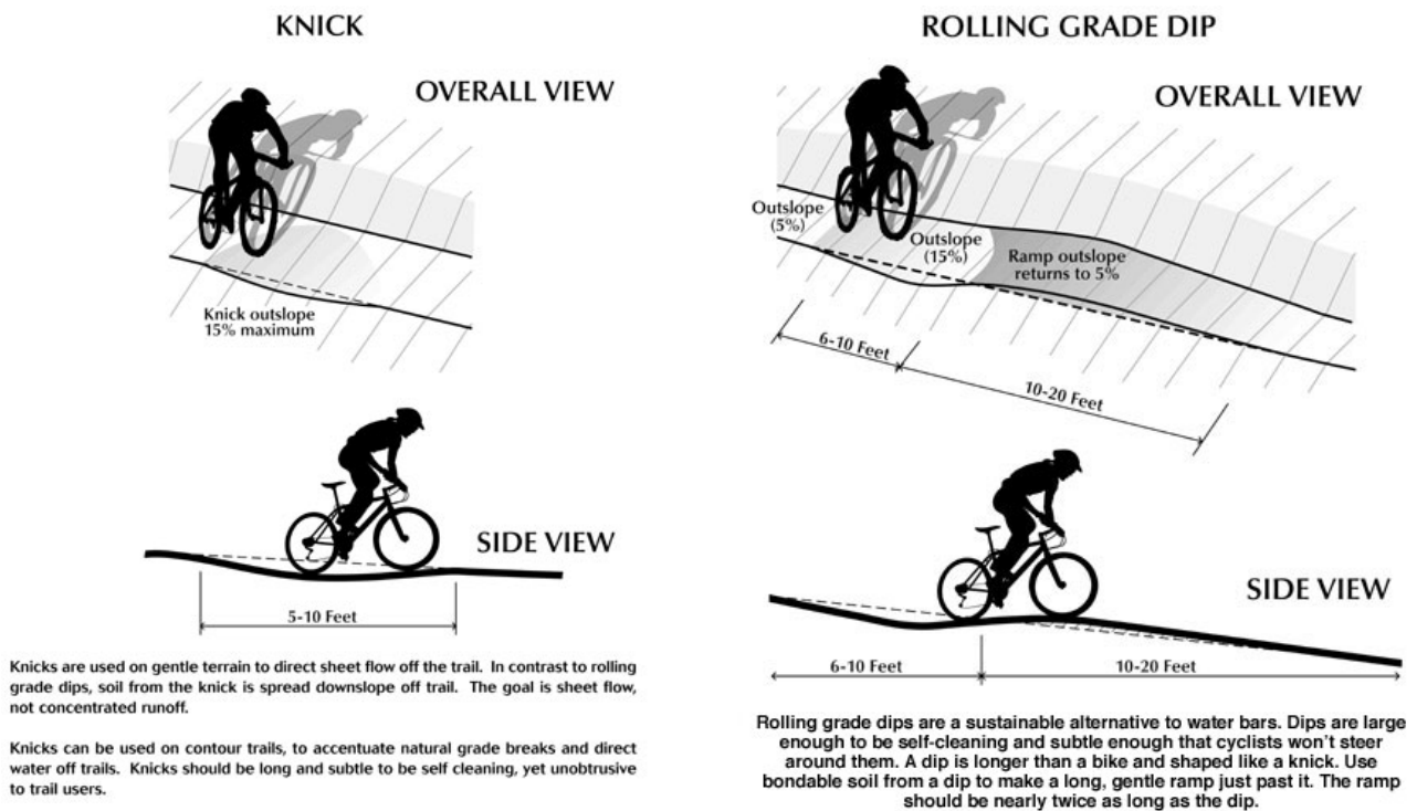
Figuur 11 Schematische weergave van 'rolling grade dips' en 'knicks'
