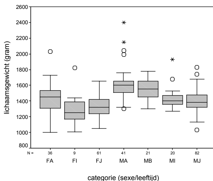
Figuur 12. Boxplot (mediaan, kwartielen en extreme waarden) van het lichaamsgewicht (in gram) voor de dood gevonden Eidereenden per categorie. Negen dieren met een borstspier conditie index van 3 zijn niet meegerekend. M=man, F=vrouw; A=adult(volwassen); B=subadult (3e en 4e winters, alleen bij mannen), I=’immature’ (2e winter), J=juveniel (1e winter).
