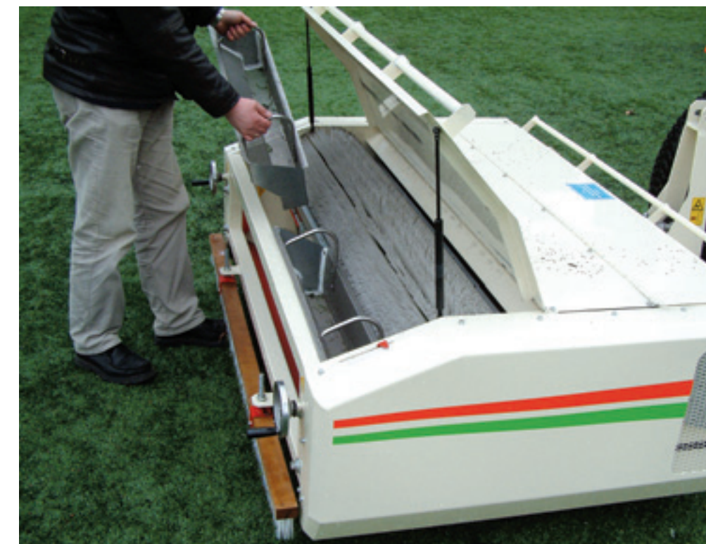
De diepteinstelling van de Hörger is nauwkeurig te regelen met draaispindels. Fijn stof wordt afgezogen en komt in twee stoffilterzakken die voor op de machine zitten. Grover vuil komt in twee groffilters die achterop zitten. De filters zijn eenvoudig leeg te maken.
