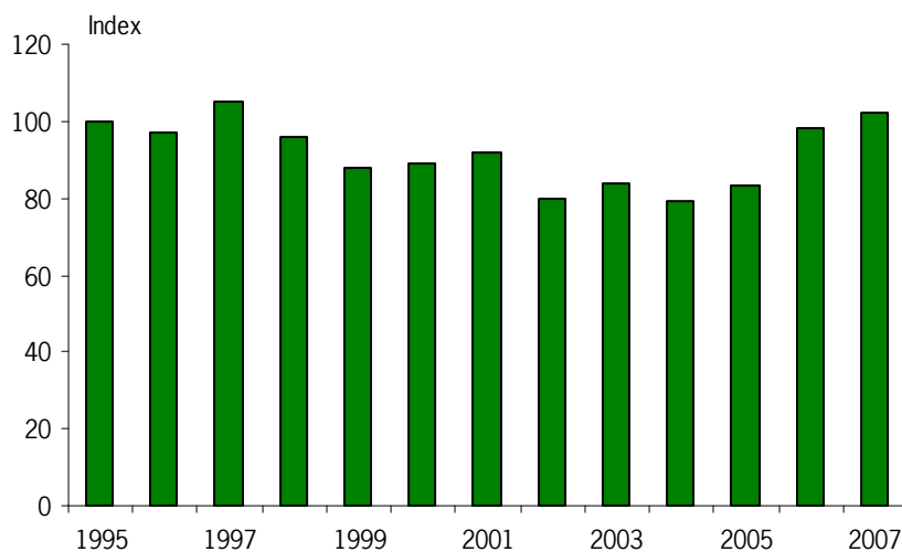
Figuur 1 Netto toegevoegde waarde per arbeidskracht, index 1994-1996 = 100
