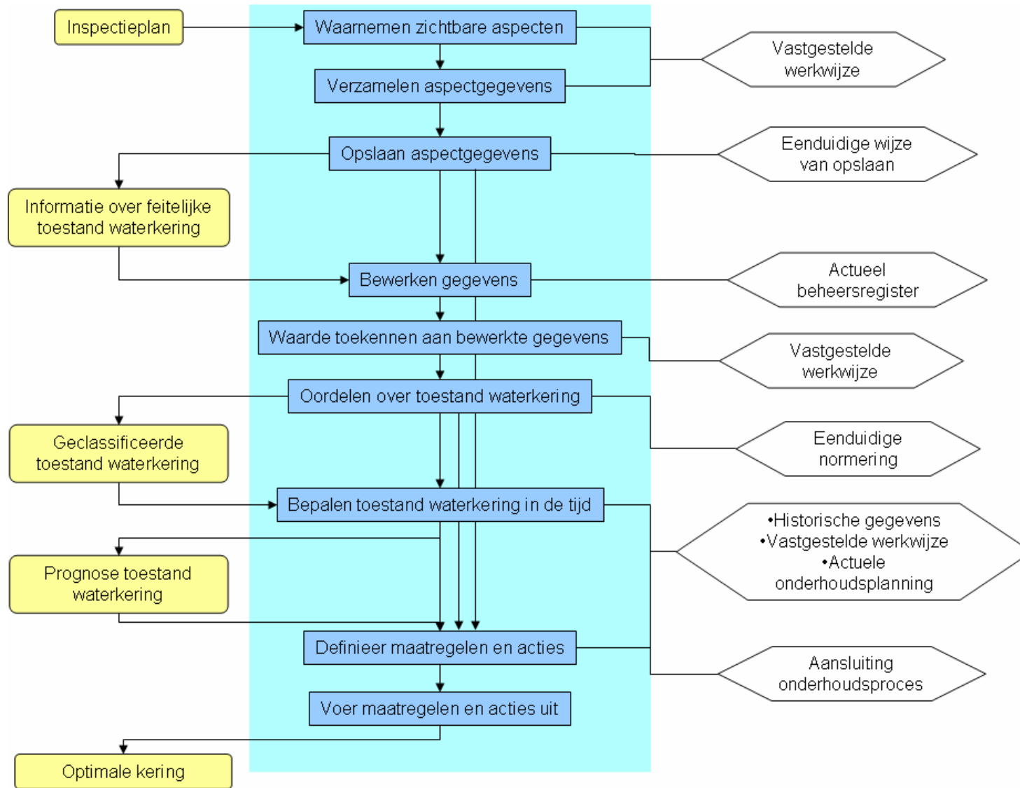
Figuur 10 Processchema inspectieproces
