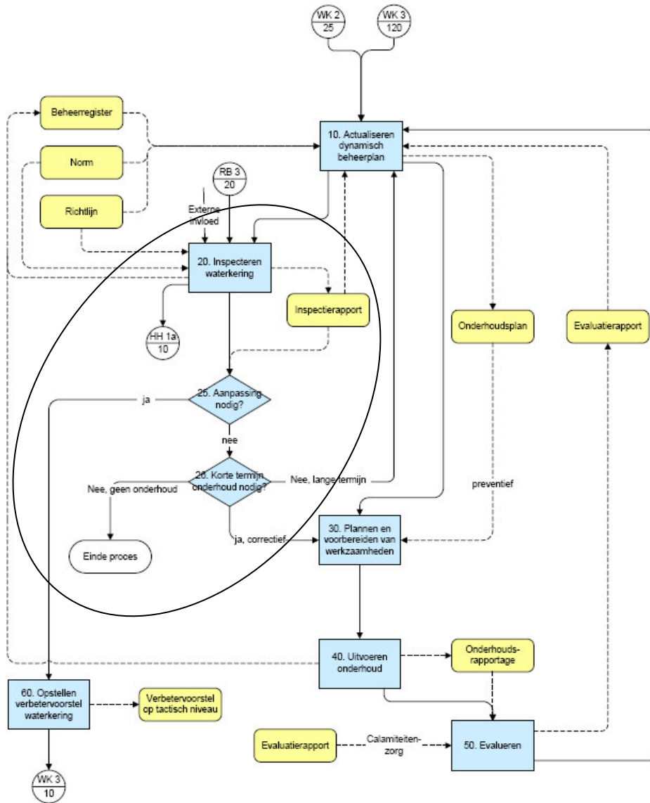
Figuur 5 Schematisering proces In stand houden waterkering (WIA): het ovaal bevat inspecties
