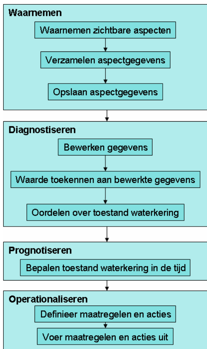
Figuur 8 Schematische weergave inspectieproces in deelprocessen en subprocessen
