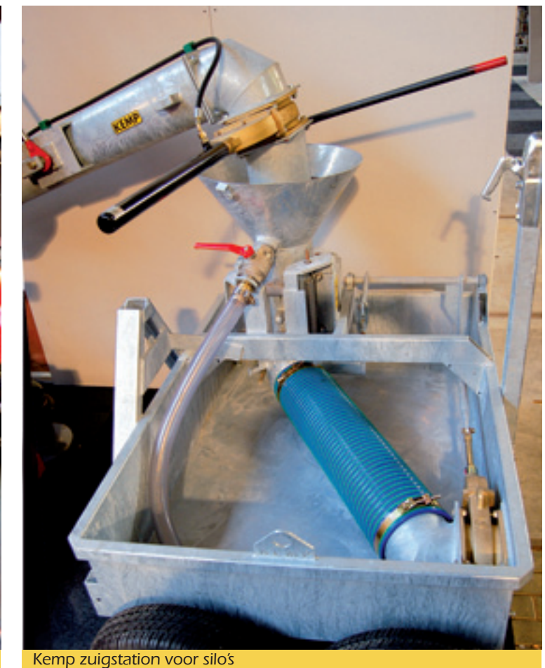
Kemp zuigstation voor silo's
