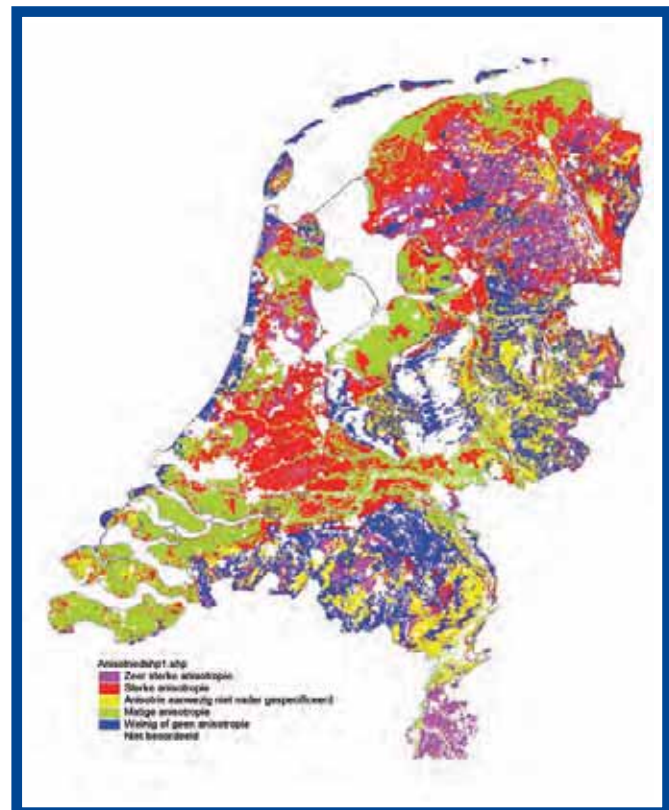
Afb. 7: Anisotropiekaart
