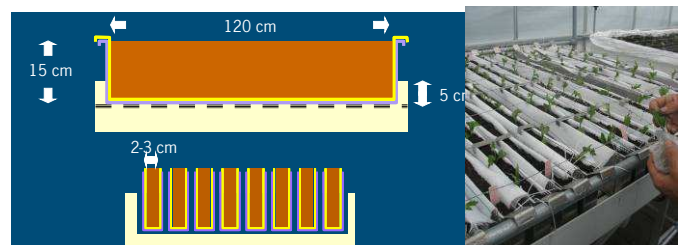
Systeem 5, Cassettebedden
