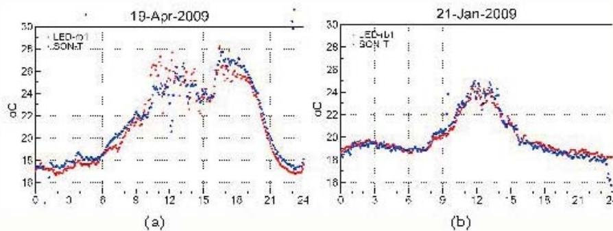
Figuur 2.3. Bladtemperatuur rd-1 en son-t behandeling bij een hoge instraling (a) en lage instraling (b).
